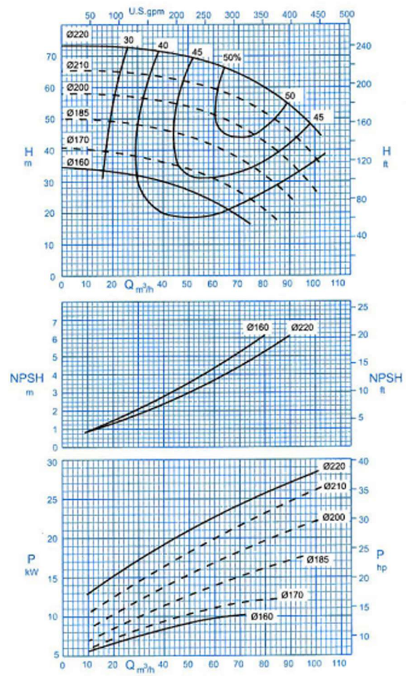
نمودار آبدهی در دور موتور ۲۹۰۰
