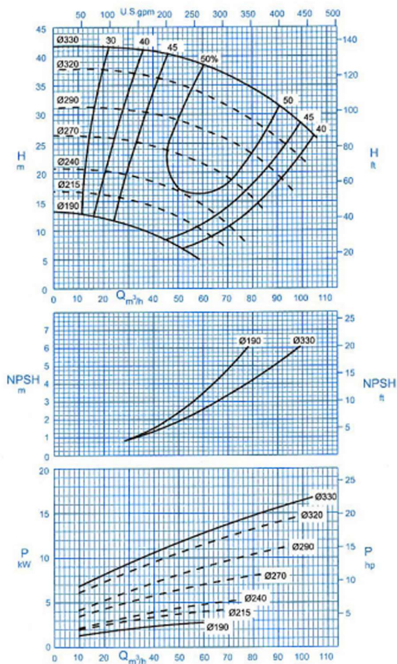
نمودار آبدهی در دور موتور ۱۴۵۰
